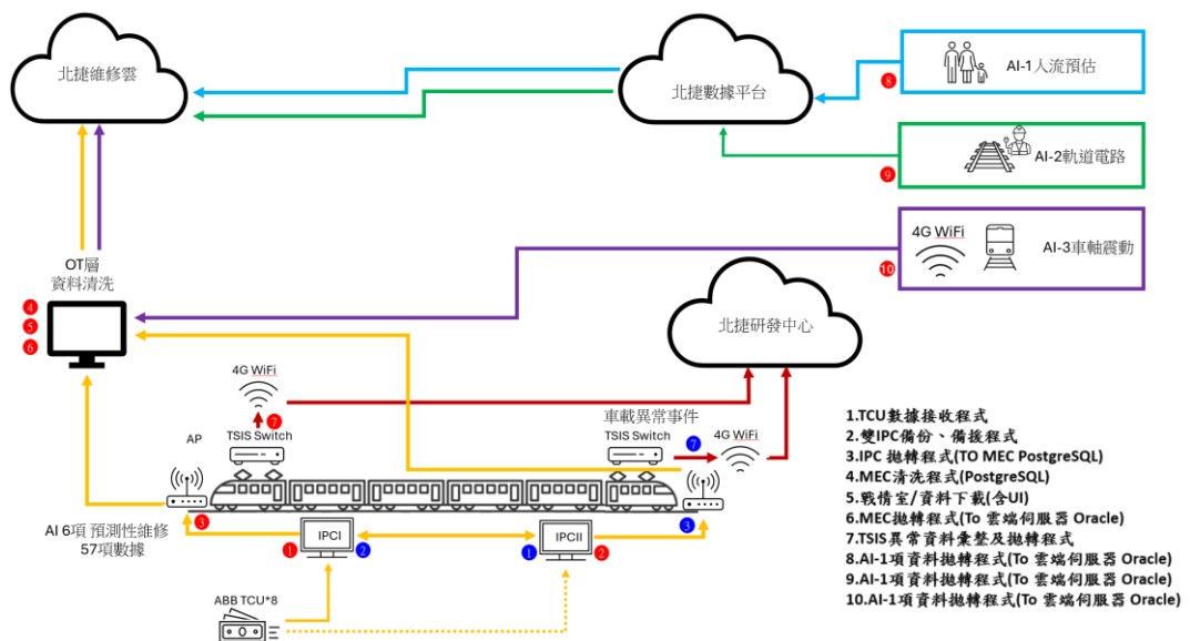
圖 1、整體架構圖
